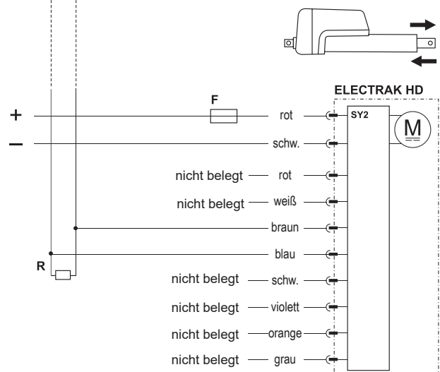
Aktuator 2 (Empfänger)
